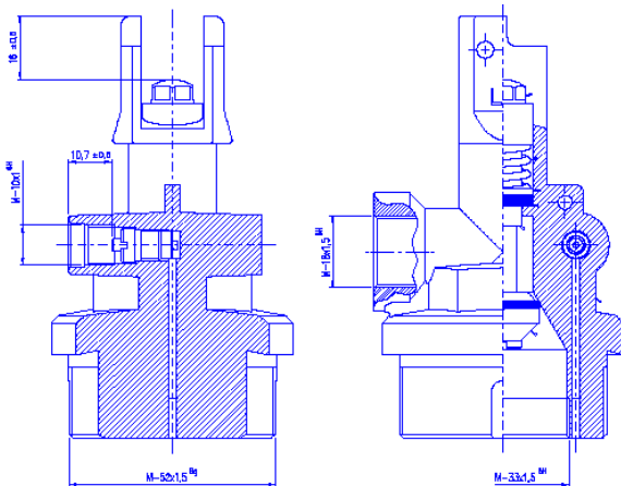
DETALLE PLANO VÁLVULA EXTINTOR PP50HDI
