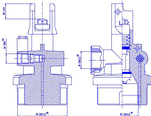
DETALLE PLANO VÁLVULA EXTINTOR PP50P
